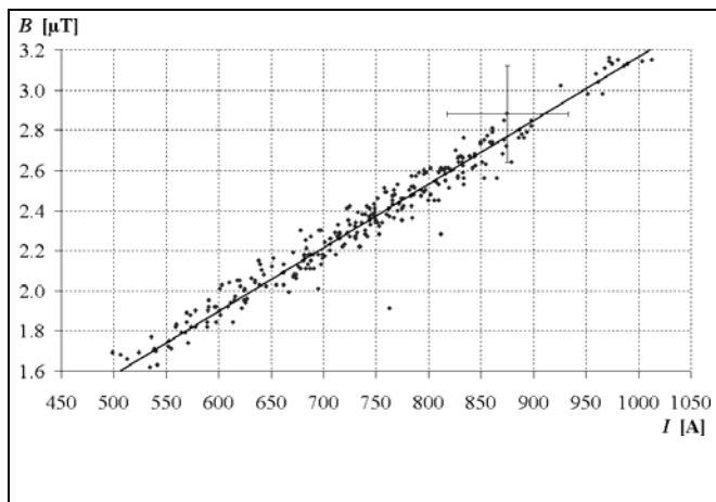
Figura 3: Relazione tra l'induzione misurata e la corrente di linea per la linea singola 356 a 380 kV.
