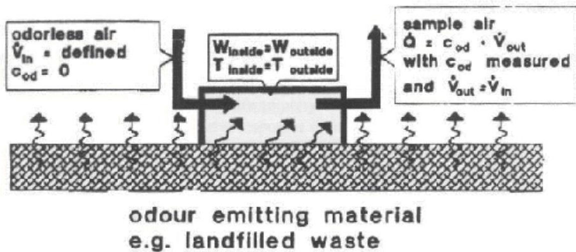
Figura 8. Schema di funzionamento di una cappa per il campionamento da superfici areali passive
