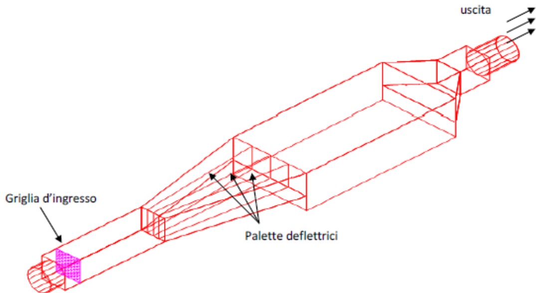
Figura 10. Esempio di vista tridimensionale di una wind tunnel
