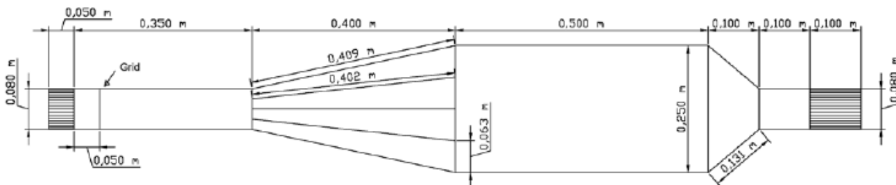
Figura 9. Esempio di pianta di una wind tunnel
