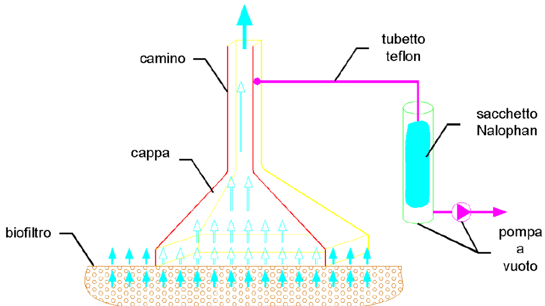
Figura 7. Schema di campionamento da sorgente areale attiva (biofiltro)
