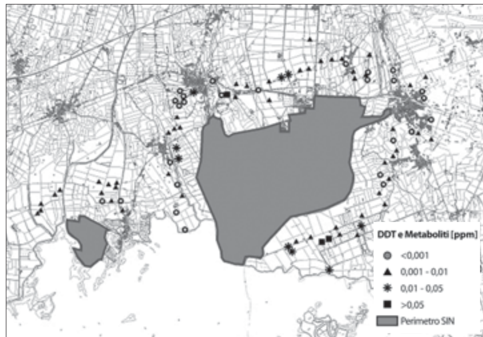
FIGURA 11. DISTRIBUZIONE SPAZIALE DI DDT E METABOLITI.
