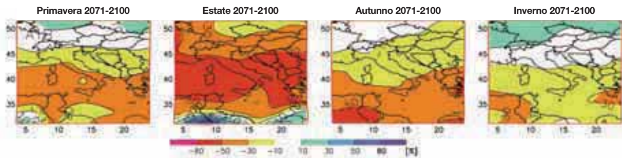
FIGURA 12. VARIAZIONE DELLE PRECIPITAZIONI ANNUALI MEDIE NEL PERIODO 2071-2100 RISPETTO AL PERIODO DI RIFERIMENTO 1961-1990 (SCENARIO SRES A1B) PREVISTO DAL MODELLO DI CIRCOLAZIONE GENERALE GFDL-CM2.1. I PANNELLI RAPPRESENTANO LA VARIAZIONE MEDIA NELLE QUATTRO STAGIONI DELL'ANNO. IL MODELLO GFDL-CM2.1 È UNO DEI 20 MODELLI UTILIZZATI NELLO STUDIO CONDOTTO DA FAGGIAN, GIORGI (2009) DA CUI È TRATTA L'IMMAGINE.
